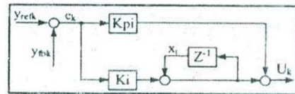
Fig. 4. Regulador PI básico.
